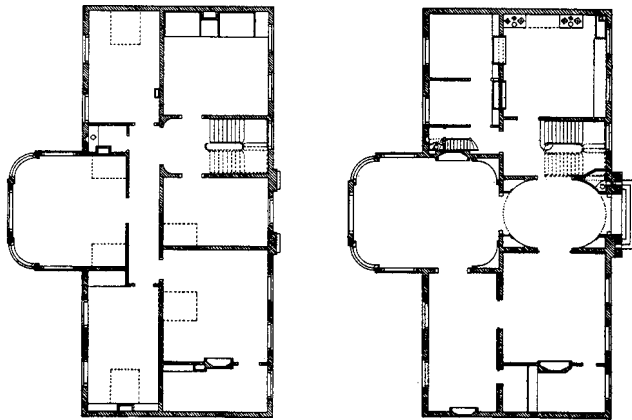
Fig. 8. PLATTEGROND VAN HET DEFINITIEVE ONTWERP, DAT SLECHTS MET KLEINE WIJZIGINGEN WERD UITGEVOERD, 1774
