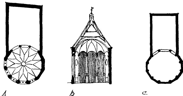
Afb. 5. — A en B. : Plattegr. en doorsnede v. d. Jerusalemskapel te Gouda (1504). — C. : Plattegr. van een fragmentarisch bewaarde onbekende kapel te Delft, later deel uitmakend van het Oude Vrouwenhuis. — Naar: Maandblad Amstelodamum.
