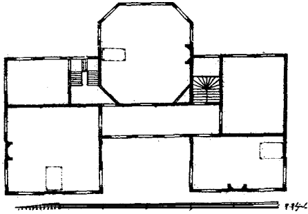
Fig. 5. VERBOUWINGSPLAN OMSTREEKS 1765, VERDIEPING Schaal 1 : 400
