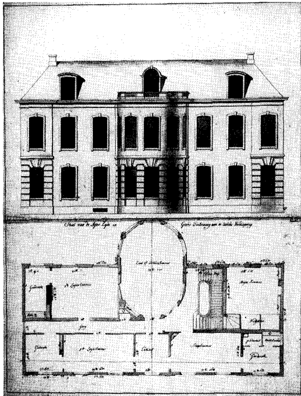
Afb. 6. ONTWERPTEKENING VOOR EEN VERBOUWING VAN HET HUIS RIJNHOF
