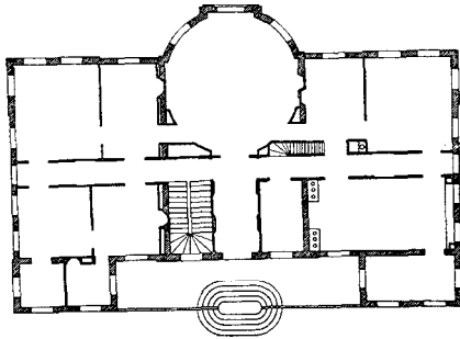
Fig. 5. VERBOUWINGSPLAN OMSTREEKS 1765, VERDIEPING Schaal 1 : 400
