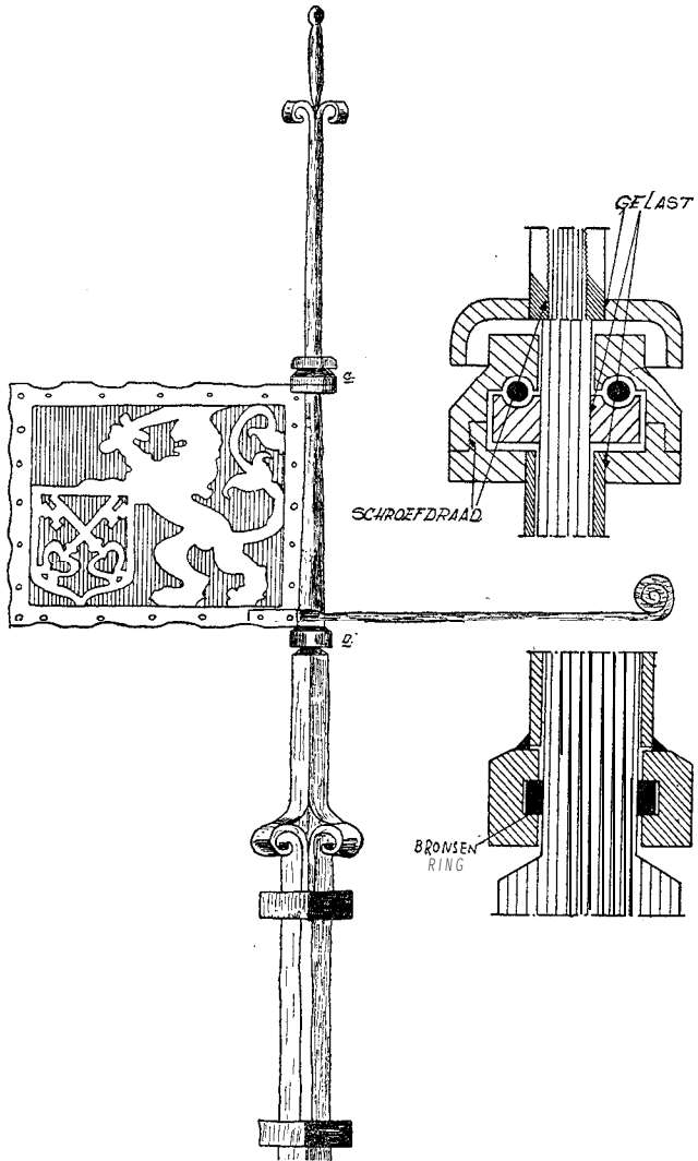
Afd. I WINDVAAN GRAVENSTEEN MET DRAAI-CONSTRUCTIE.
