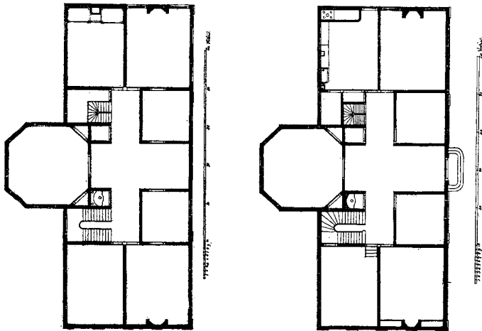
Fig.3. VERBOUWINGSPLAN OMSTREEKS I 765, BEGANEGROND EN VERDIEPING Schaal 1 : 400
