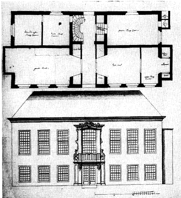
Afb. 1. ONTWERPTEKING VOOR DE VERNIEUWING VAN RHIJNHOF Ongesigneerd, ongedateerd ± 1760.
