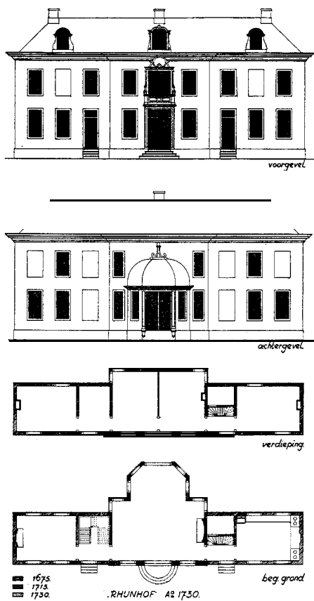
Fig. 2. RHIJNHOF NA DE VERBOUWING IN 1730 NAAR EEN OPMETING VAN J. S. CREUTZ Schaal 1 : 400
