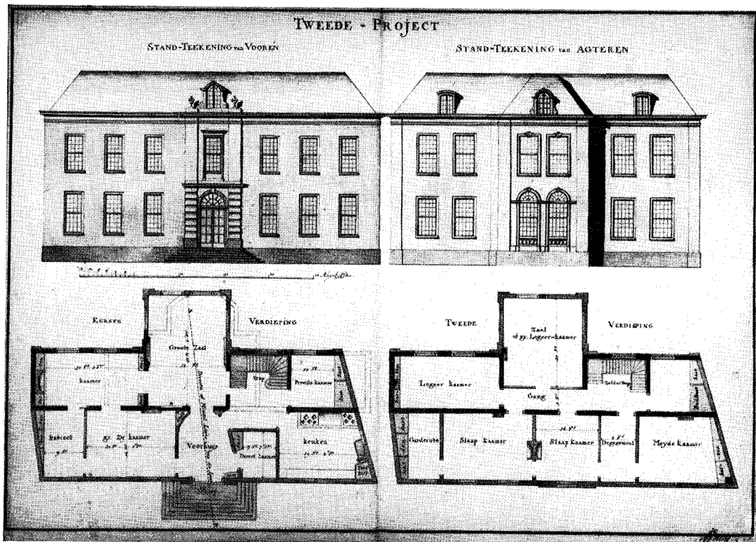
Afb. 7. „TWEDE PROJECT” VOOR DE VERBOUWING VAN RHIJNHOF; J. S. CREUTZ, ongedateerd, ± 1773.
