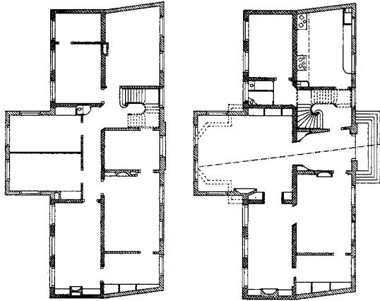
Fig. 7. PLATTEGROND VAN HET „DERDE PROJECT“, gesigneerd door J. S. CREUTZ, ± 1773 Schaal 1 : 400
