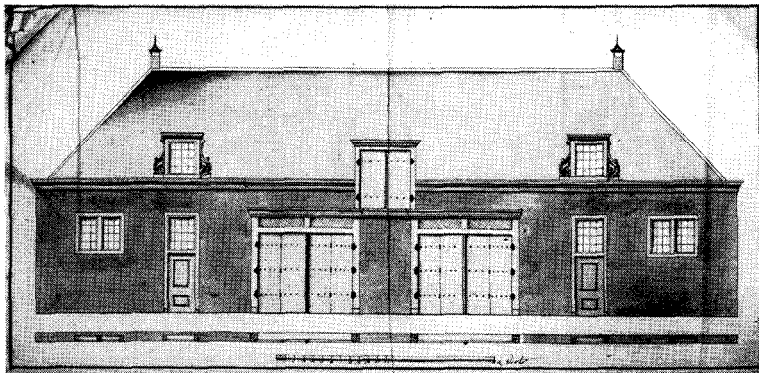
Afb.2. ONTWERPTEKING VOOR HET THANS NOG BESTAANDE KOETSHUIS, 1767. Ongesigneerd, gevel aan de straatzijde.
