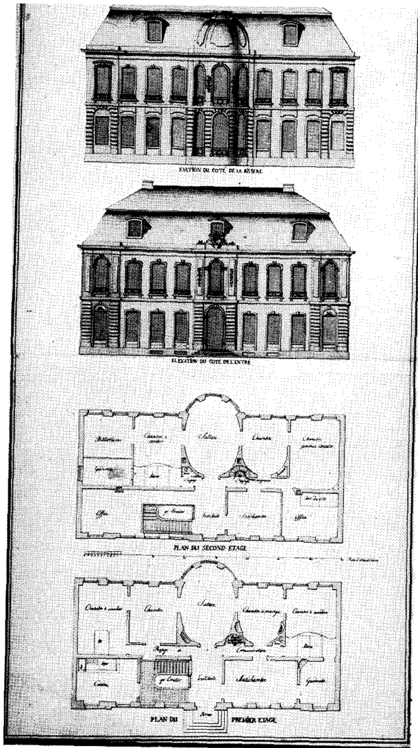
Afb. 4. ONTWERPTEKENING VOOR EEN GEHEEL NIEUW RHIJNHOF Ongesigeneerd en ongedateerd; vermoedelijk J. S. CREUTZ ±1773.
